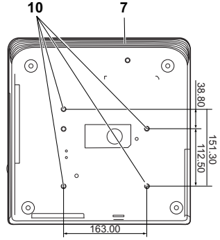
底視圖
